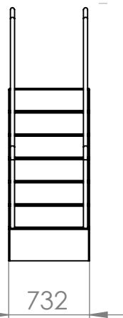
SCALE 1 : 20
