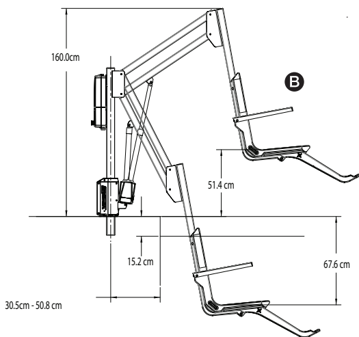
B SIDE VIEW VISTA LATERAL VUE DE CÔTÉ SEITENANSICHT VISTA LATERALE
